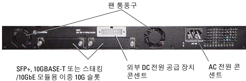
그림 1-9. PC7024P 및 PC7048P 후면 패널
